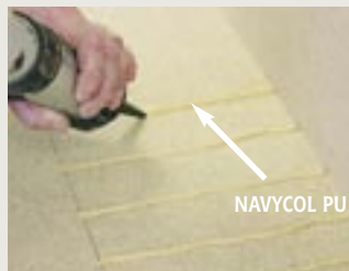
1 - Après pose à blanc du parquet, collage cordon avec NAVYCOL
